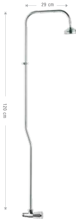
539MS Gruppo doccia monoacqua con colonna doccia. Wall mtg. single water shower set with shower column.
