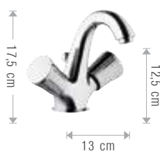
395MS Monoforo lavabo con scarico. Single hole basin set with pop-up waste. CR
