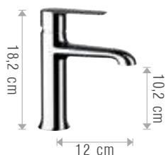
380AR Miscelatore monocomando lavabo senza scarico e senza foro sul corpo. Single-lever basin mixer without waste and without body hole. CR FIN ( .14 .08 )
